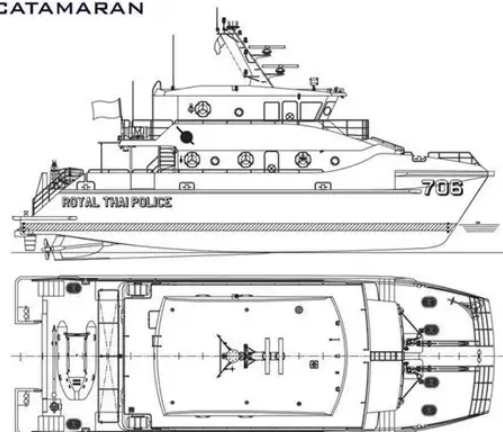
23M. CATAMARAN
